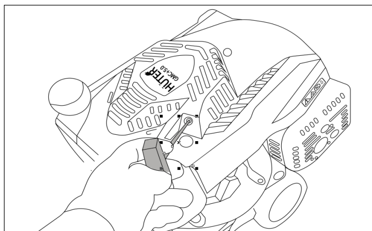
Рис. 15. Ручка стартера
