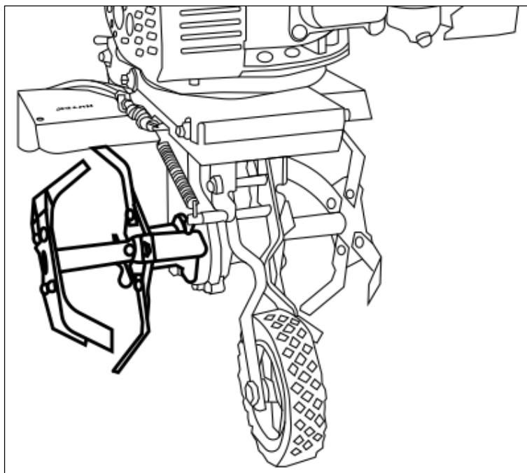
Рис. 7. Установка фрез
