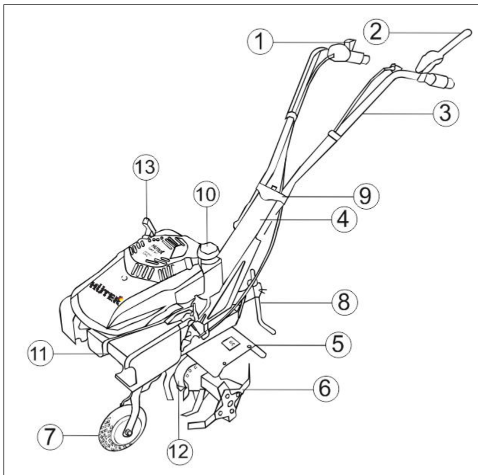
Рис. 1. Общий вид
